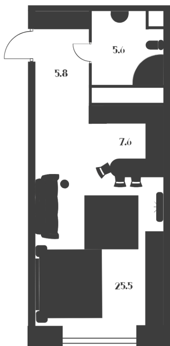
ПЛАН ЭТАЖА, 5 ЭТАЖ
