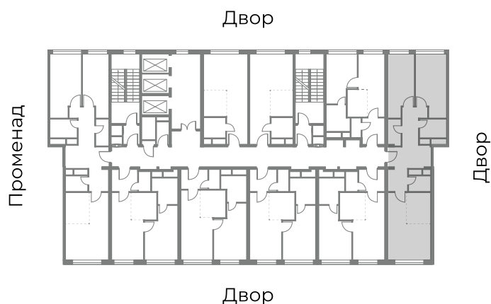
ПЛАН ЭТАЖА, 18 ЭТАЖ
