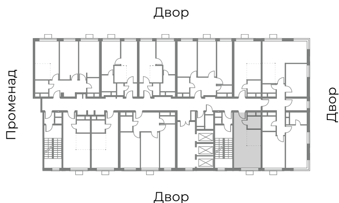
ПЛАН ЭТАЖА, 16 ЭТАЖ
